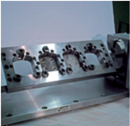
Mechanische Vorrichtung als Spannbrücke.
