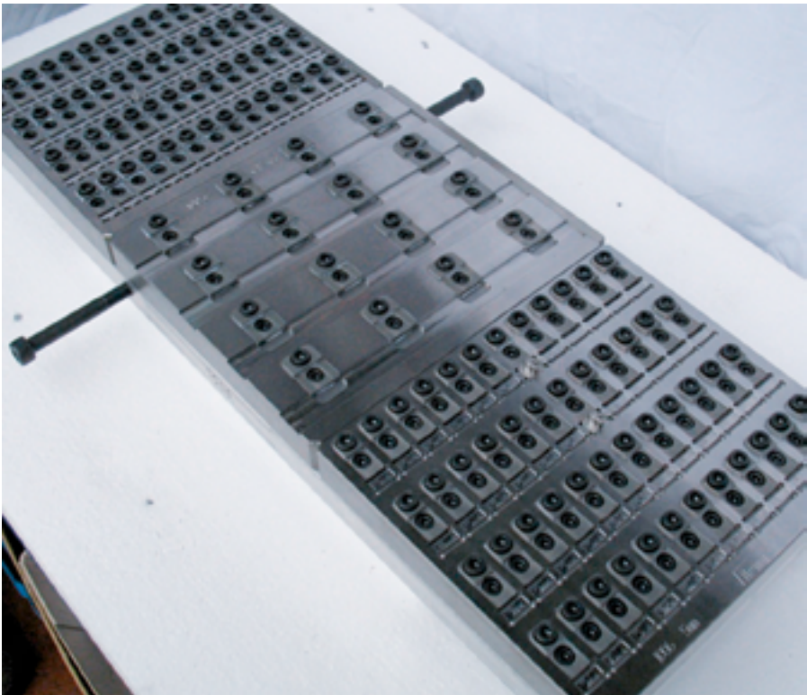
Mechanische Vorrichtung zur Mehrfachspannung von Kleinteilen.
